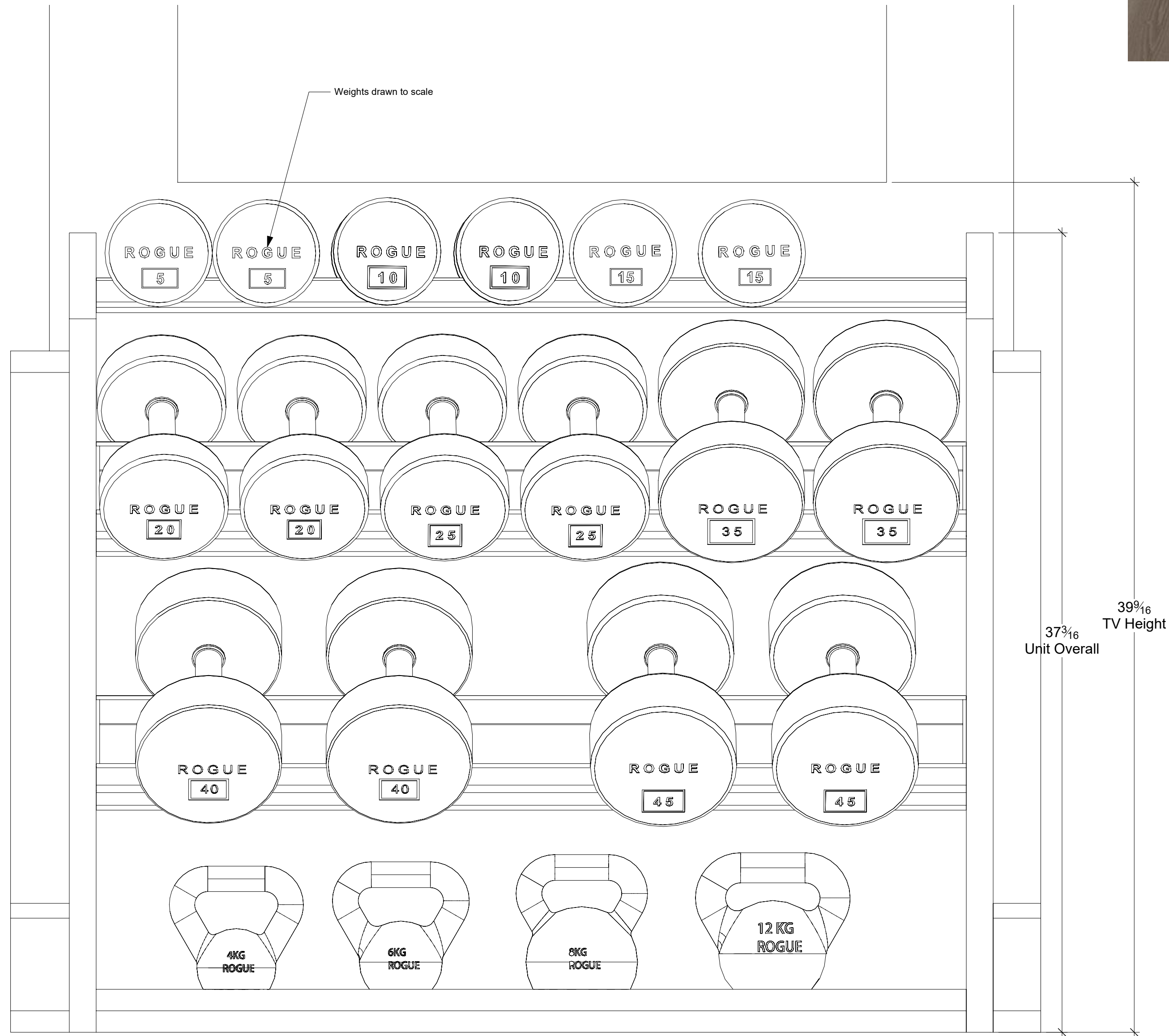
7 Front Scale: 3" = 1'-0"
