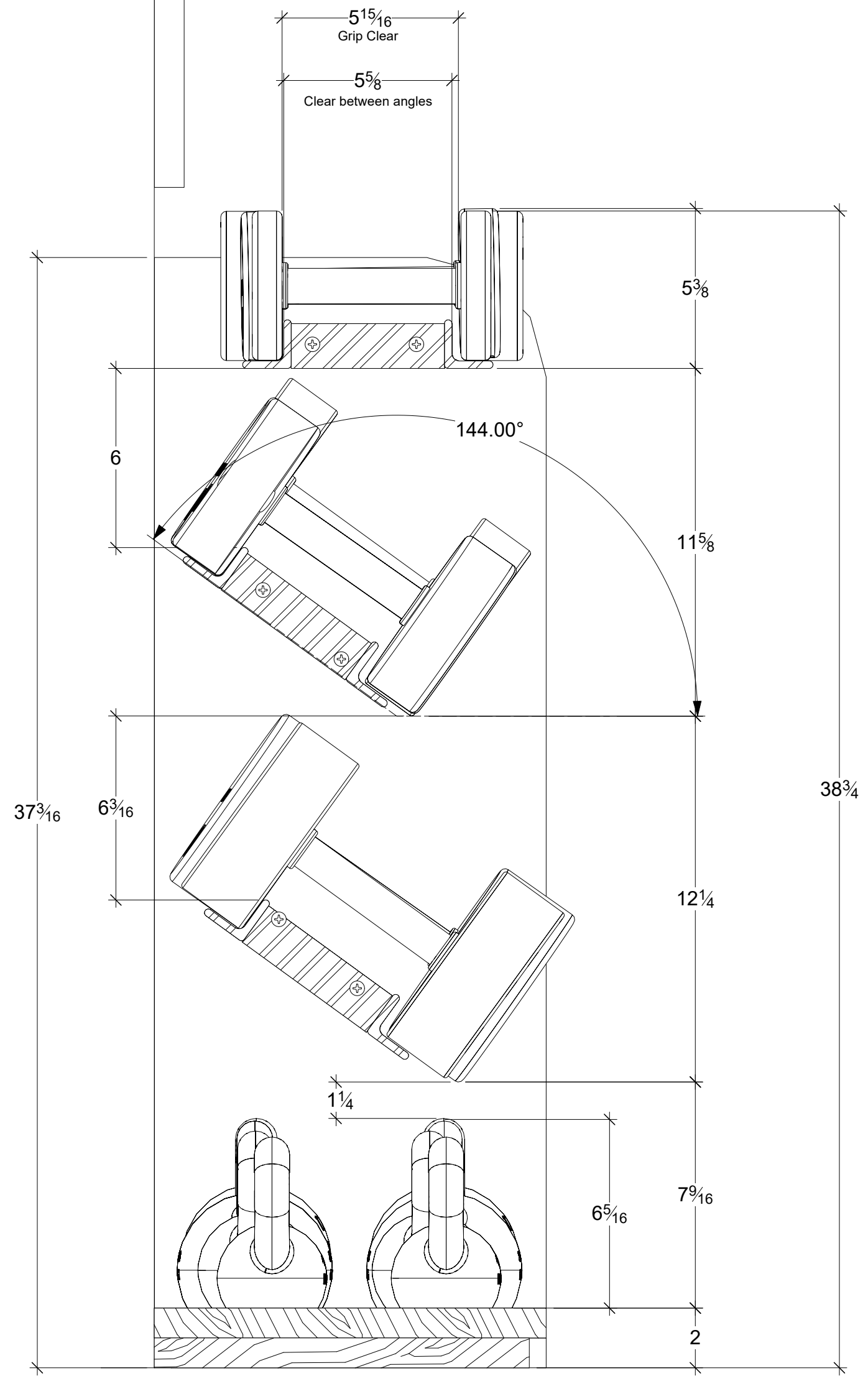
6 Side Scale: 3" = 1'-0"
